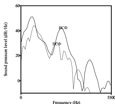
Рисунок 5 – Оригінальні криві спектрів співочих голосних [а] у виконанні Д. Гнатюка та Б. Гмирі
