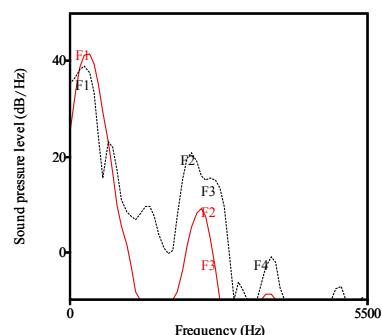
Рисунок 3 – Оригінальні криві спектрів співочого та мовленнєвого голосних [и] у виконанні Р. Майбороди
